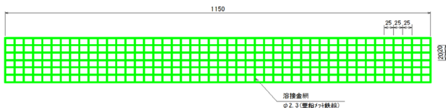
フラット金網枠 詳細図
