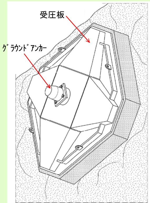
④グラウトアンカー施工、受圧板設置
